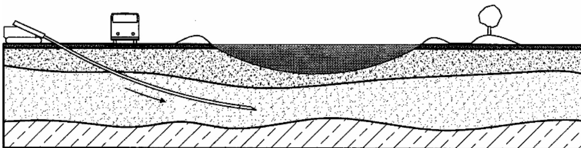
Rys.1) Przewiert pilotażowy
