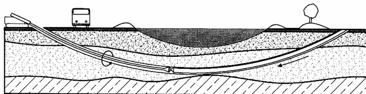
Rys.3) Przeciąganie rurociągu
